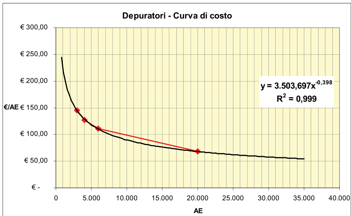
Figura 9 - Curva di costo per impianti di depurazione con potenzialità compresa tra 1.000 e 20.000 AE
