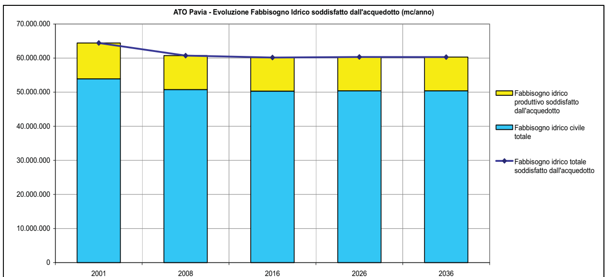
Figura 3 - Evoluzione del fabbisogno idrico soddisfatto dall'acquedotto nel periodo 2001-2036
